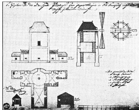
Plán větrného mlýna ve Štrampouchu zhotovený pro markýze de Trazegnies roku 1820
